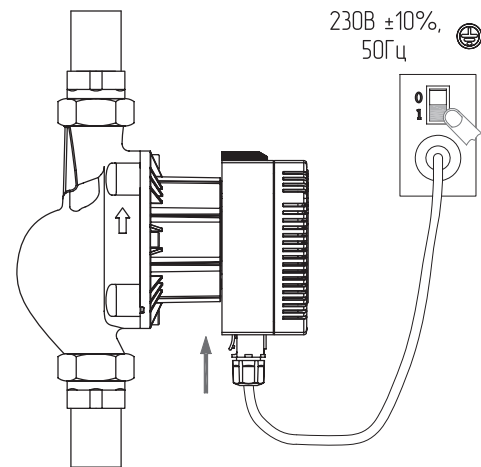
Рис. 40 Электроподключение насоса
