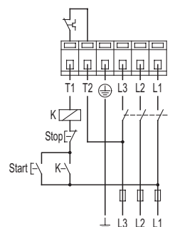
Рис. 20 Трехфазный без нейтрального провода
