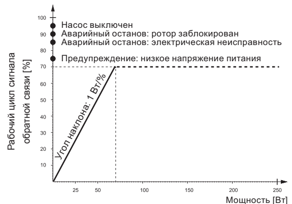
Рис. 30 Профиль ШИМ-сигнала обратной связи
