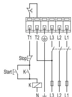
Рис. 21 Трехфазный с нейтральным проводом
