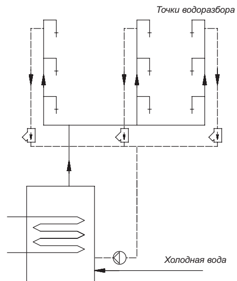
Рис. 13 Многоконтурная схема рециркуляции горячей воды
