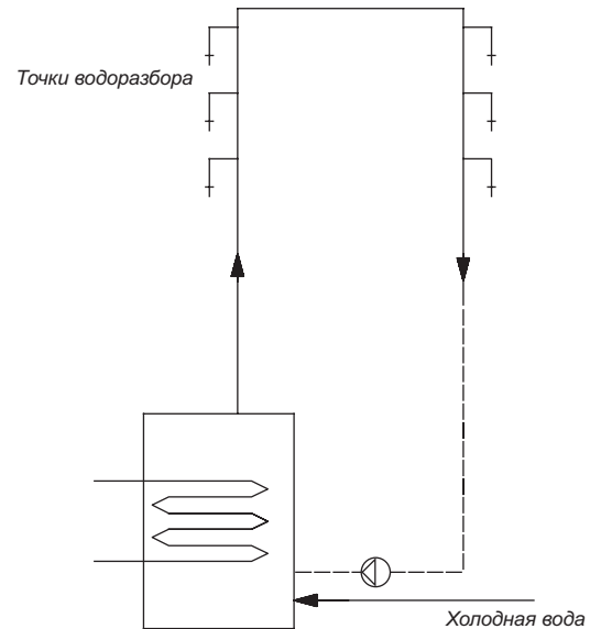
Рис. 12 Одноконтурная схема контура рециркуляции горячей воды
