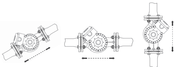
Рис. 18 Возможные положения клеммной коробки
