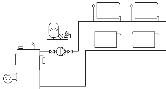
Рис. 25 Однотрубная система отопления
